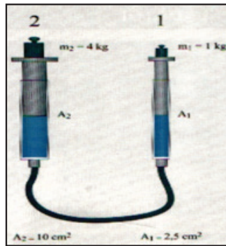
Шематски приказ огледа који је уједно и модел хидрауличне машине
