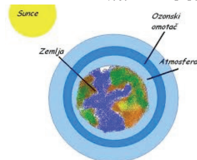
Озонски омотач Земље је оштећен
