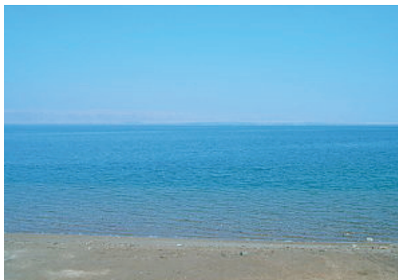
Мртво море, најсланије језеро у свету
